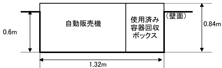
【配置図】
